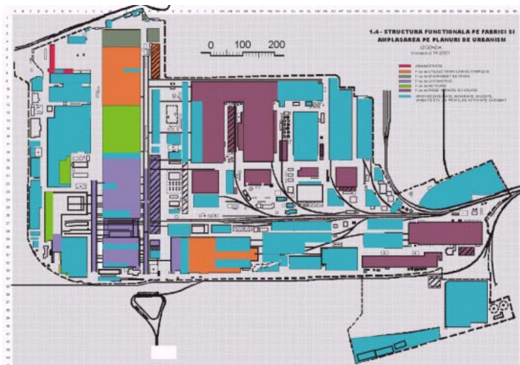
Fig. 1: Plan – Structura funcțională a uzinei
